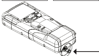
Extern filter Onderdeelnr.: SST-WTF-001
